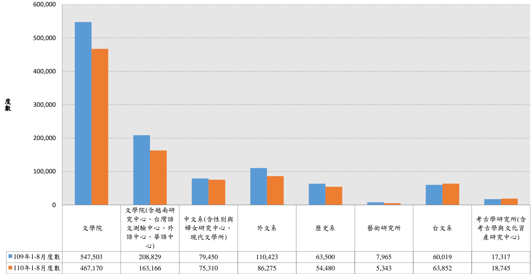
文學院110年（1~8月）相較於109年電費使用度數圖
