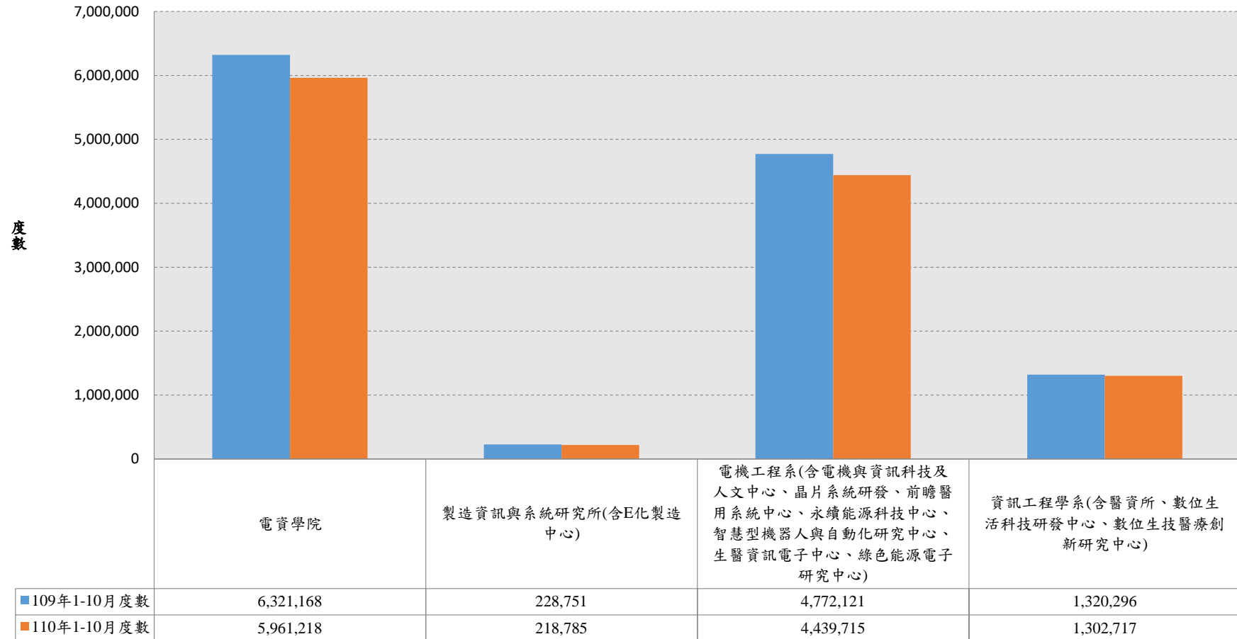
電資學院110年（1~10月）相較於109年電費使用度數圖
