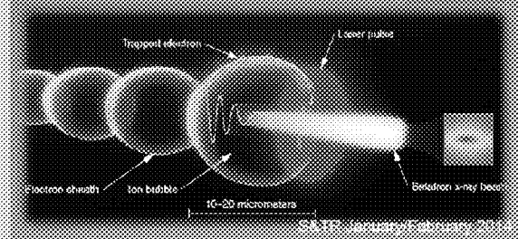
能源物理與超快技術實驗室- Laser-driven betatron x-ray source
